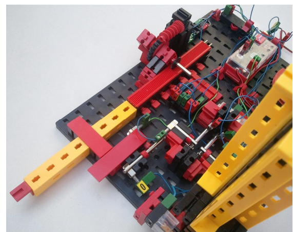
Abb. 9: Blick auf den Starttaster und die auf „4“ herausgezogene Zählstange
