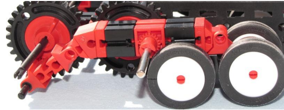
Abb. 18: Das IchBinZweiFahrwerke-Fahrwerk mit zwei Z30 nebeneinander, eingefahren ...
