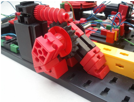
Abb. 8: Der Zählmotor
