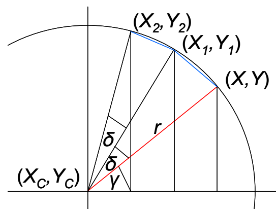
Abb. 3: Annäherung des Kreisbogens über Kreissehnen zum Winkel \delta
