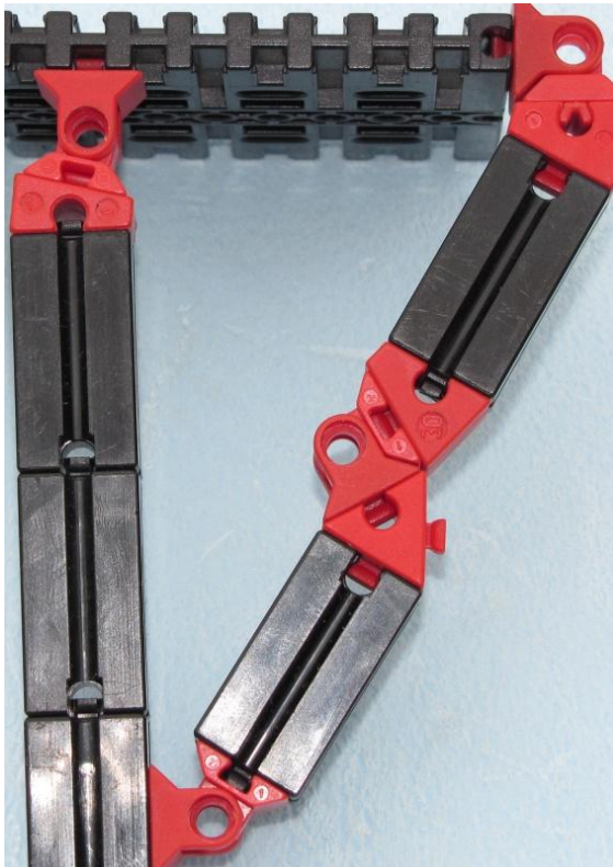
Abb. 2: ein überstrecktes Kniegelenk als Verriegelung des eigentlichen Fahrwerkbeins
