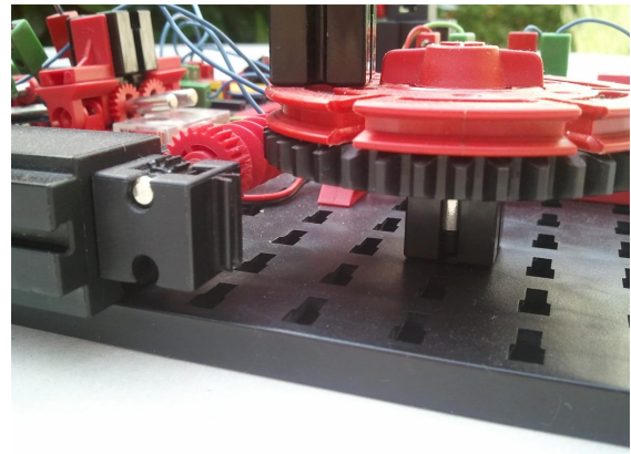
Abb. 3: Lagerung des Exzenter
