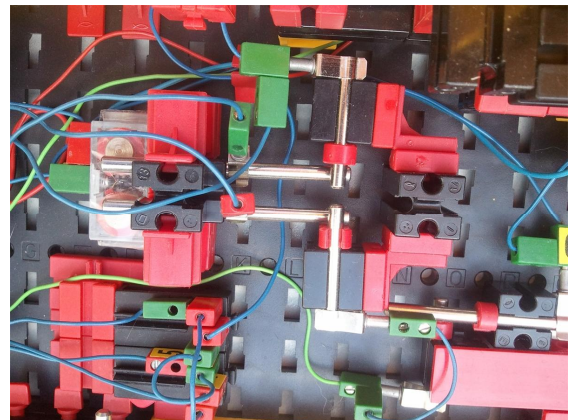
Abb. 4: Das Selbstbau-Relais
