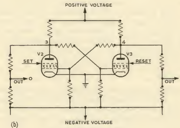
FIG. 2/15. Flip-flop circuits
