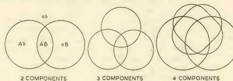
FIG. 15/1. Venn diagrams
