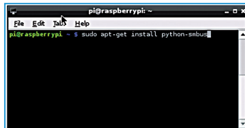
Bild 4. LXTerminal.
