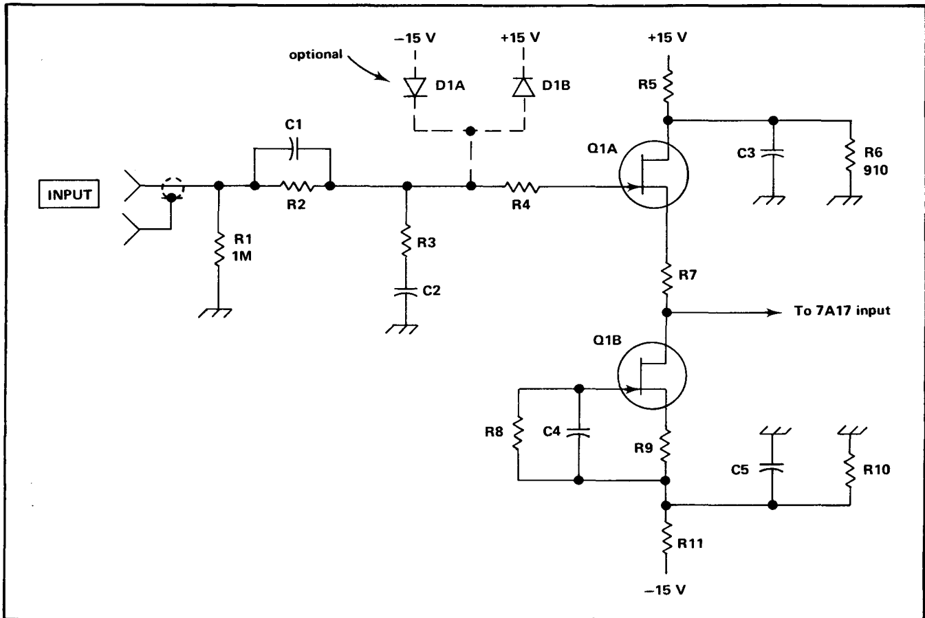
Fig. 3. FET Amplifier.
