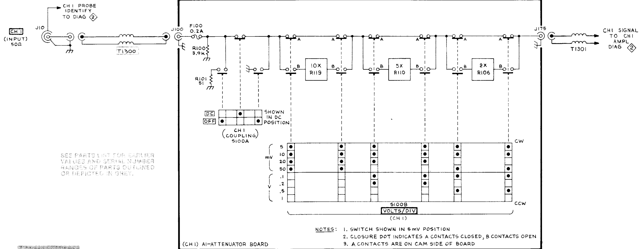
CH 1 ATTENUATOR
