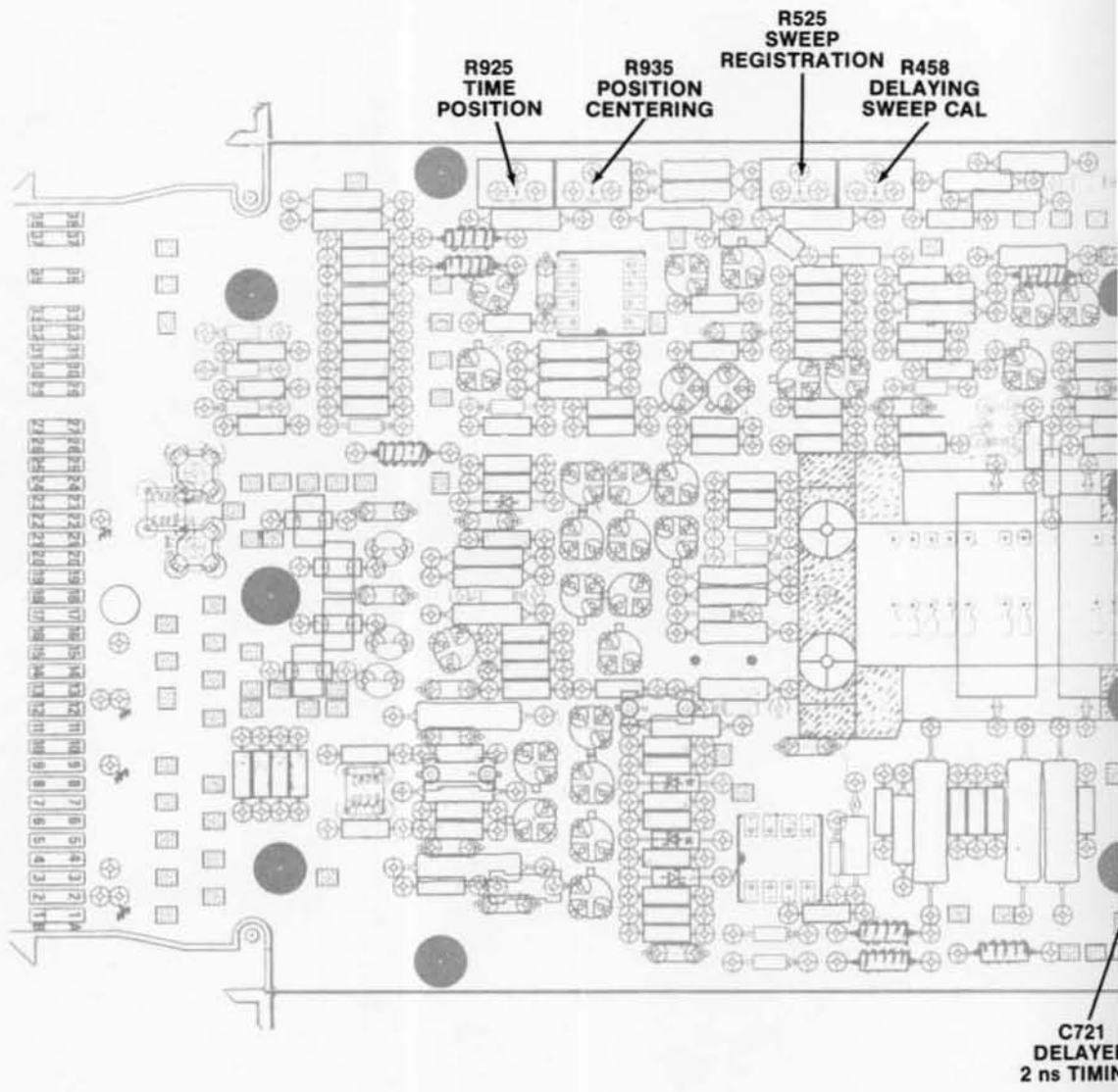
Fig. 8-18. Sweep
