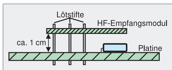
Bild 8: Die Montage des Empfangsmoduls auf der Platine
