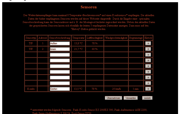
Bild 5: Auf der Seite „Sensoren“ erfolgt die Konfiguration und die Anmeldung der Wettersensoren.
