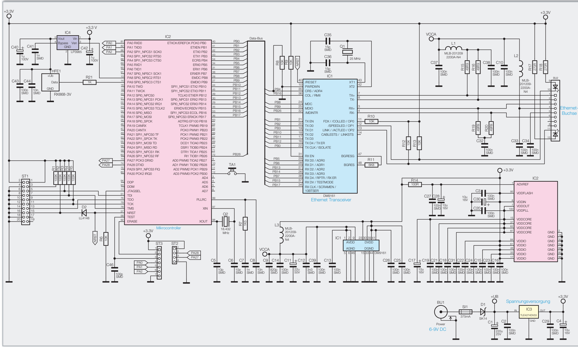
Bild 6: Das Schaltbild des Wetterdatenempfängers
