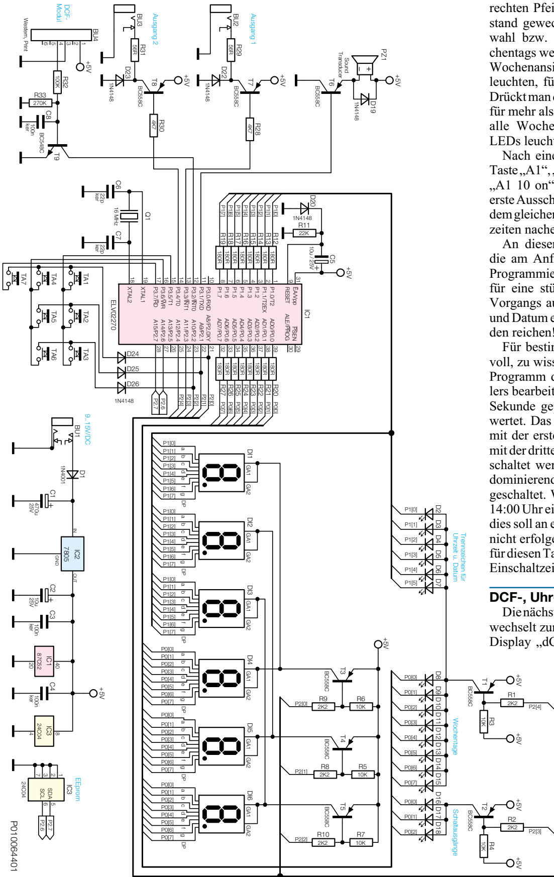
Bild 2: Schaltbild des DCF-Schaltmoduls
