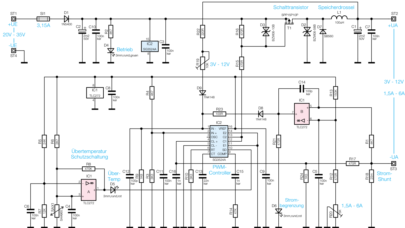
Bild 1: Schaltbild des DC/DC-Leistungskonverters
