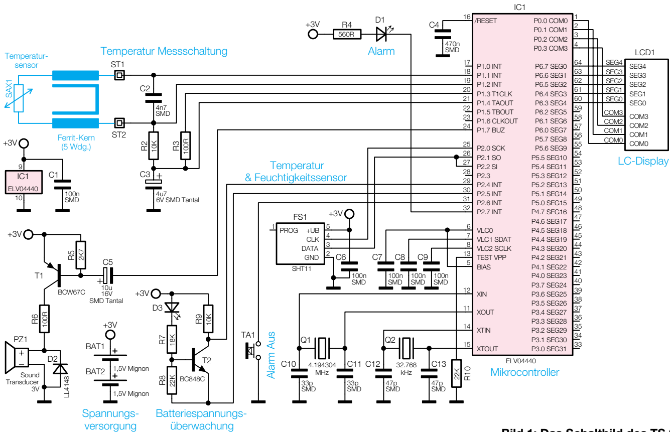
Bild 1: Das Schaltbild des TS 2
