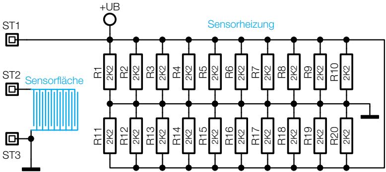
Bild 4: Schaltbild der Regensensorplatine
