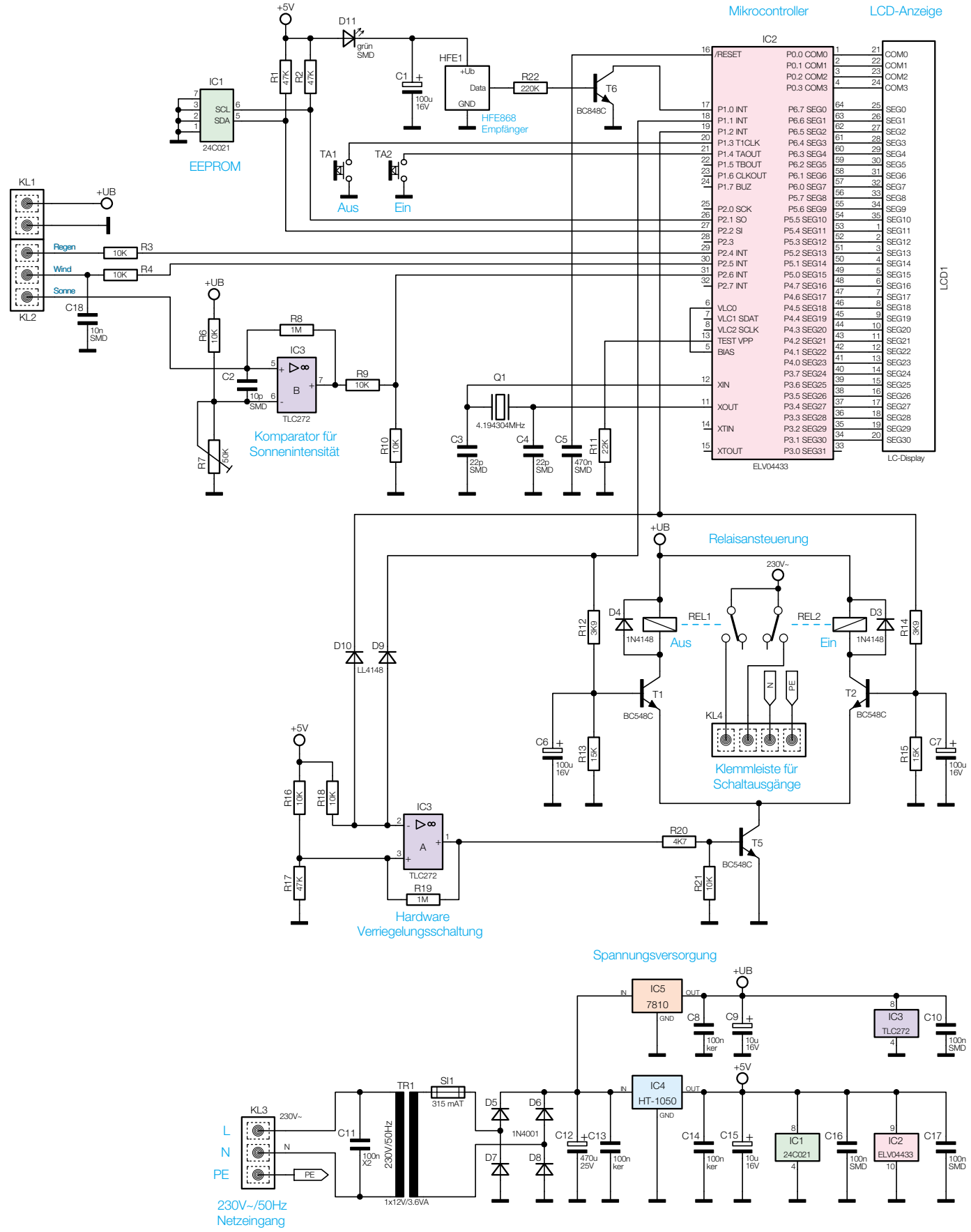
Bild 2: Schaltbild der Steuereinheit
