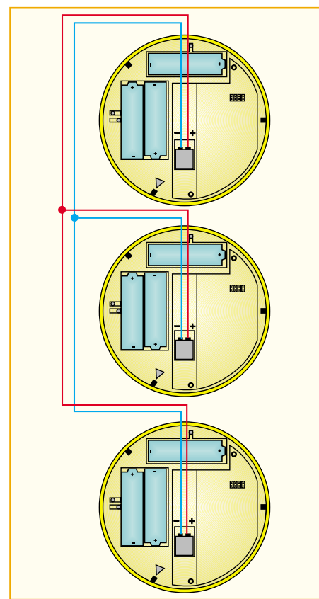
Bild 8: Besitzt der Rauchmelder eine Zweidraht-Schnittstelle, lässt er sich mit baugleichen Geräten ganz einfach vernetzen.
