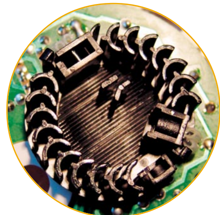
Bild 5: Die heute gängigste Form der Messkammer lässt den enormen Entwicklungsaufwand ahnen.
