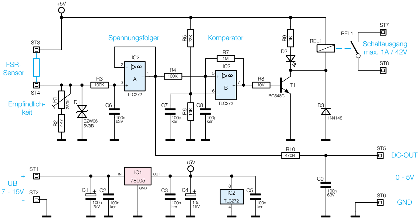
Bild 3: Schaltbild des FSR®-Drucksensors FSR 1
