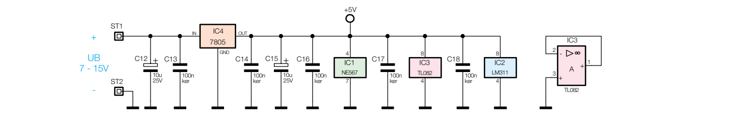
Bild 1: Schaltbild des Video-Detektors
