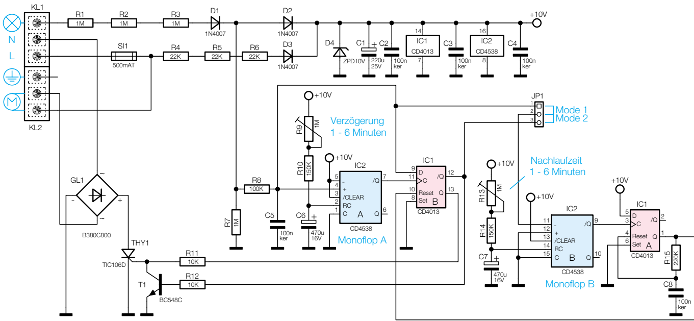
Bild 2: Schaltbild der Lüfter-Nachlaufsteuerung
