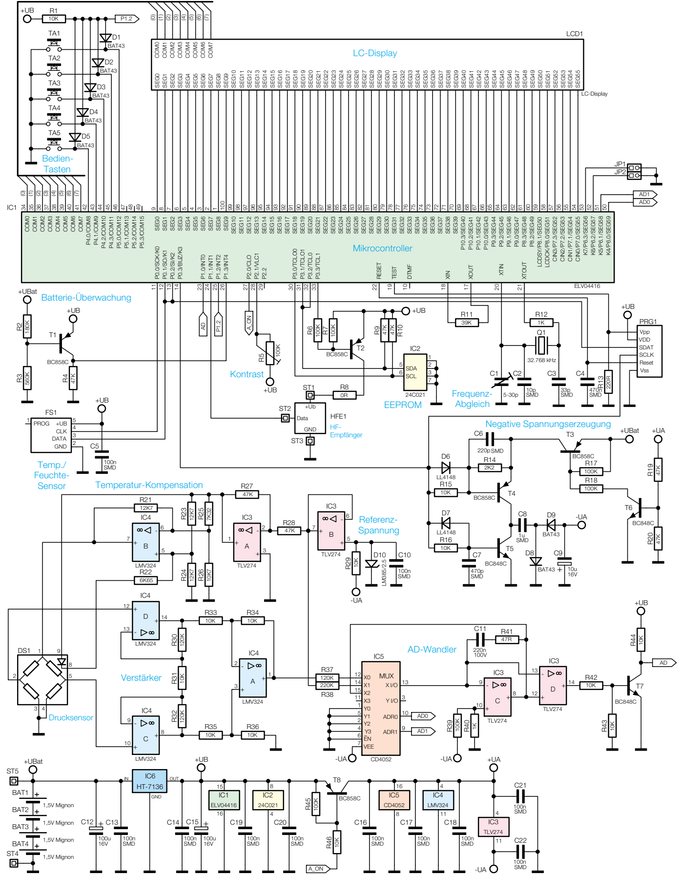
Bild 9: Schaltung der Kombi-Wetterstation WS 200
