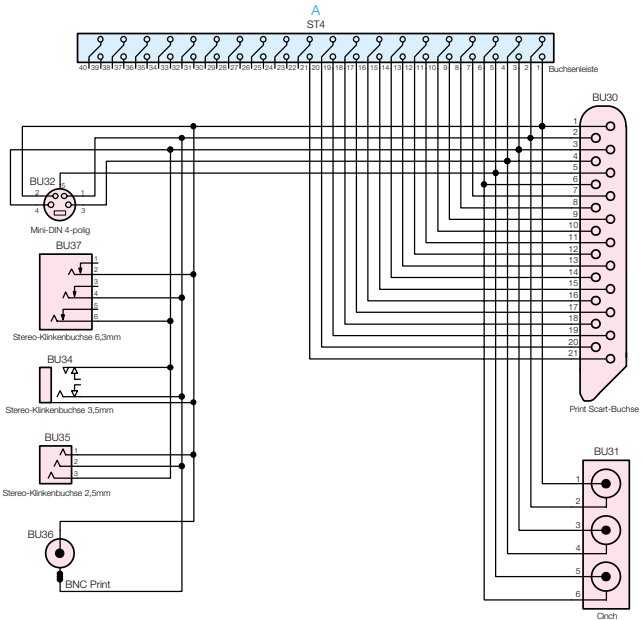
Bild 10: Schaltbild der Audio-/Video-Adapterplatine PCK 100-AV
