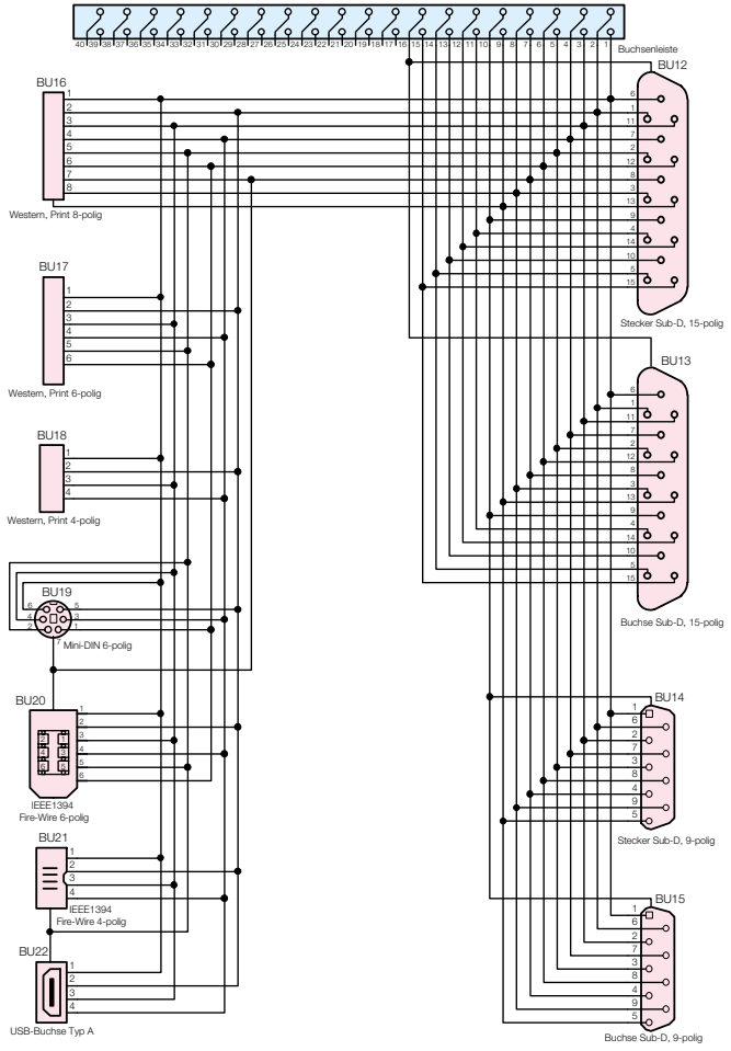
Bild 9: Schaltbild der PC-Adapterplatine PCK 100-PC
