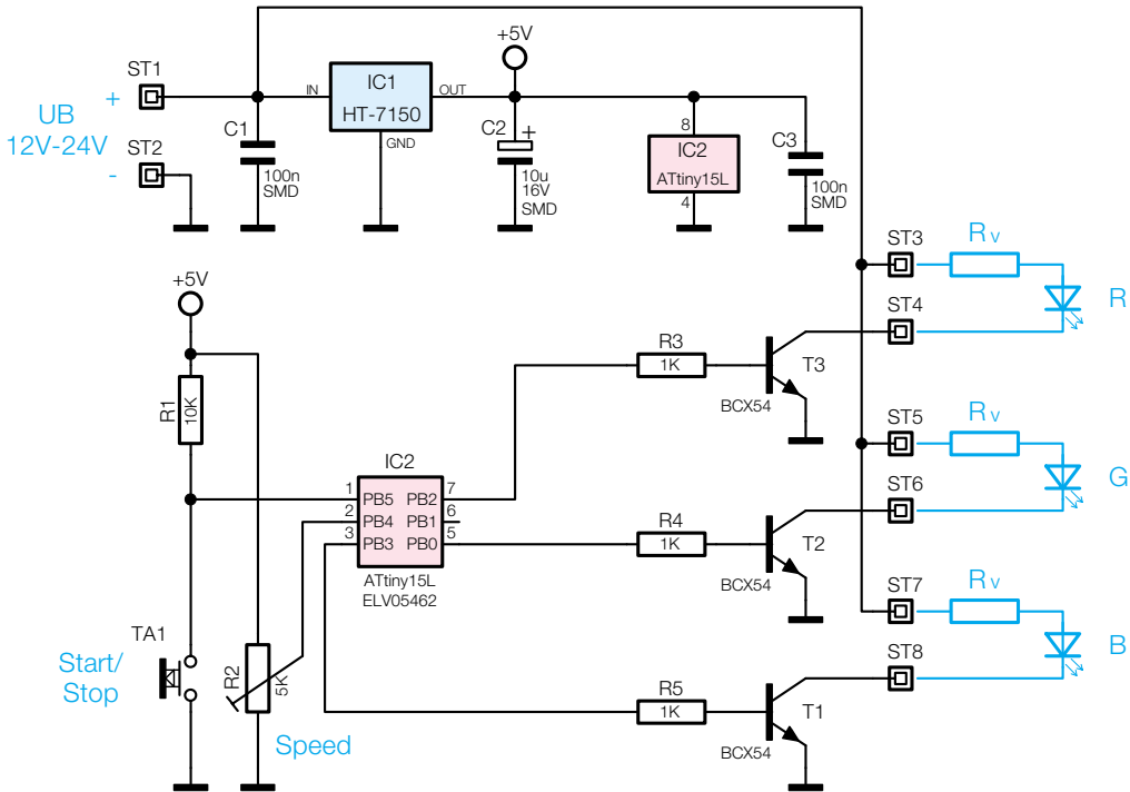
Bild 6: Schaltbild des RGB-Farbwechslers
