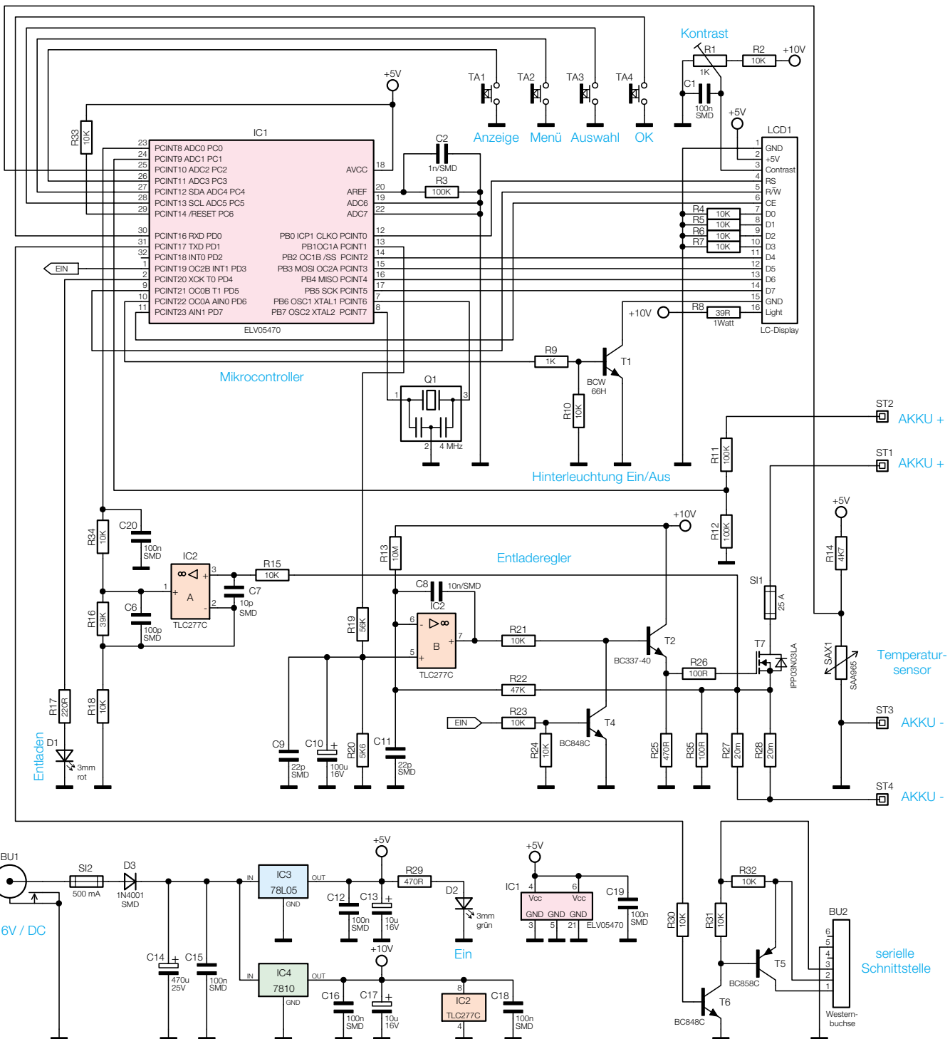
Bild 3: Schaltbild des Hochstrom-Entlade-Testgerätes HET 20
