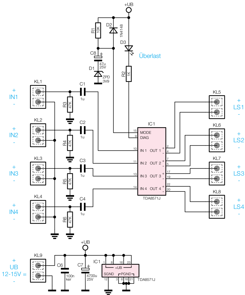
Bild 1: Schaltbild des Verstärkers V 40
