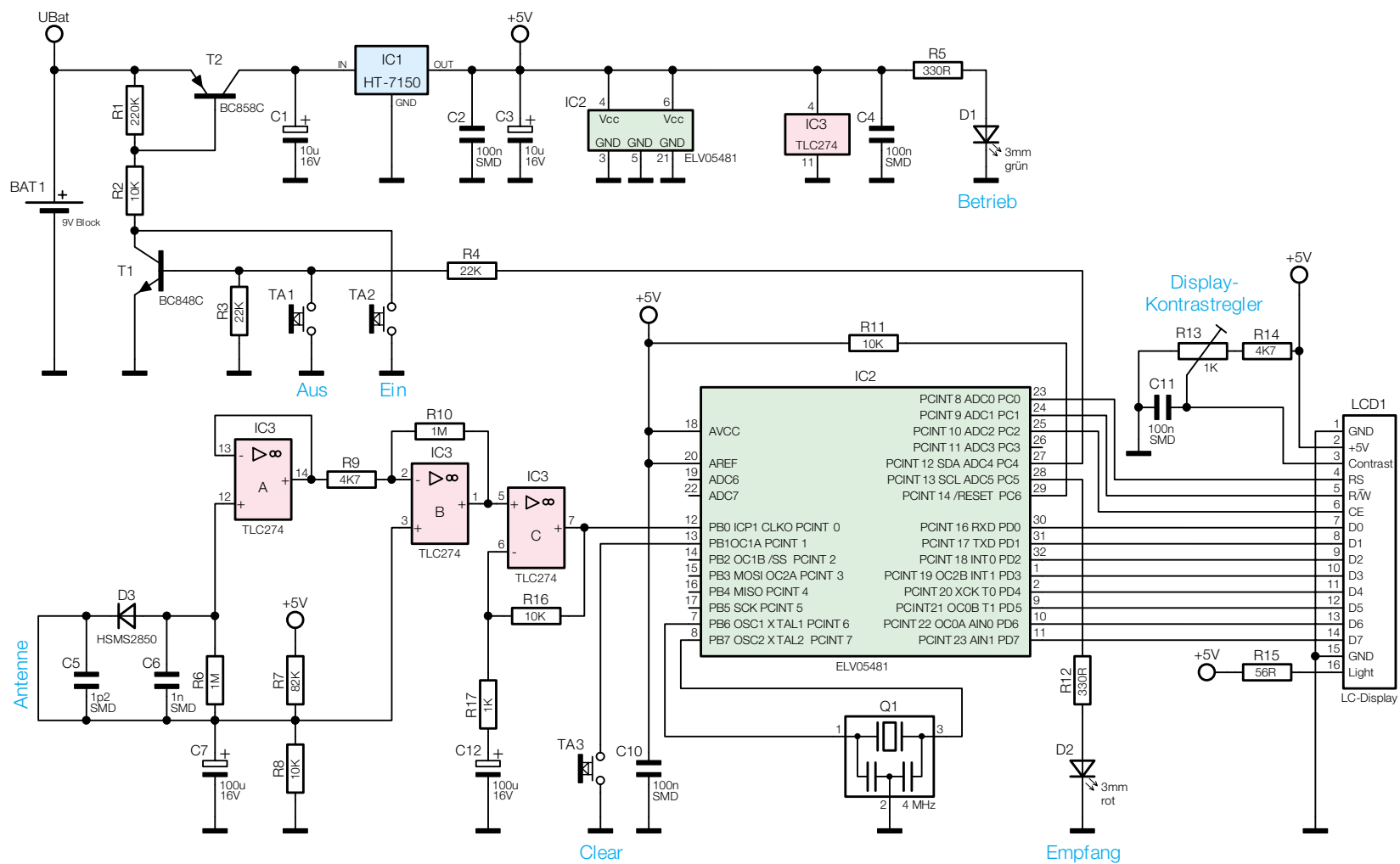
Bild 1: Schaltbild des Diagnose-Tools FS20 DT
