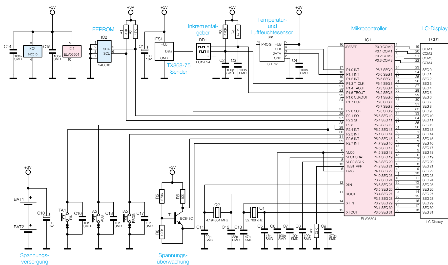
Bild 1: Schaltbild des Funk-Hygrostaten FS20 HSG
