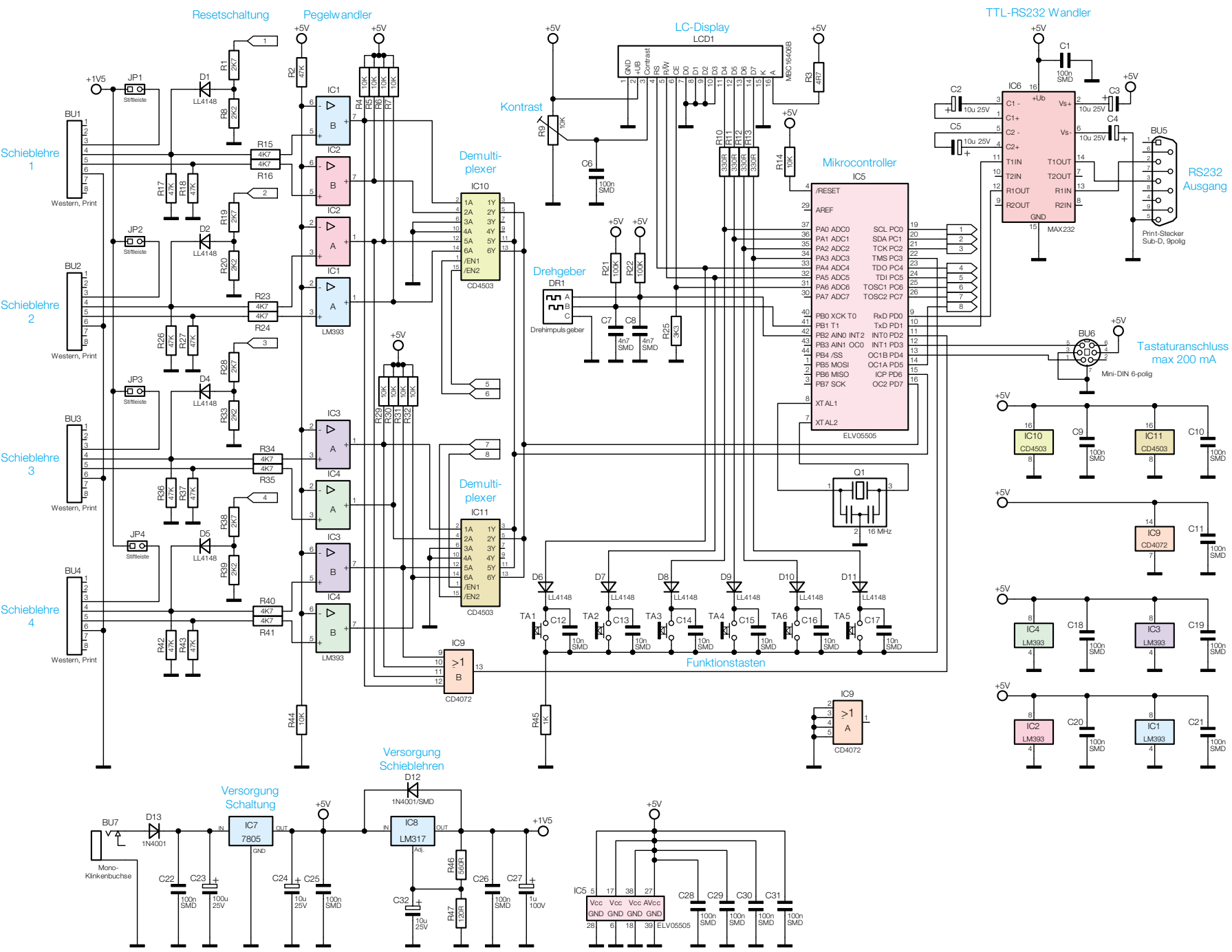
Bild 6: Schaltung der Schiebellehreneinzeile
