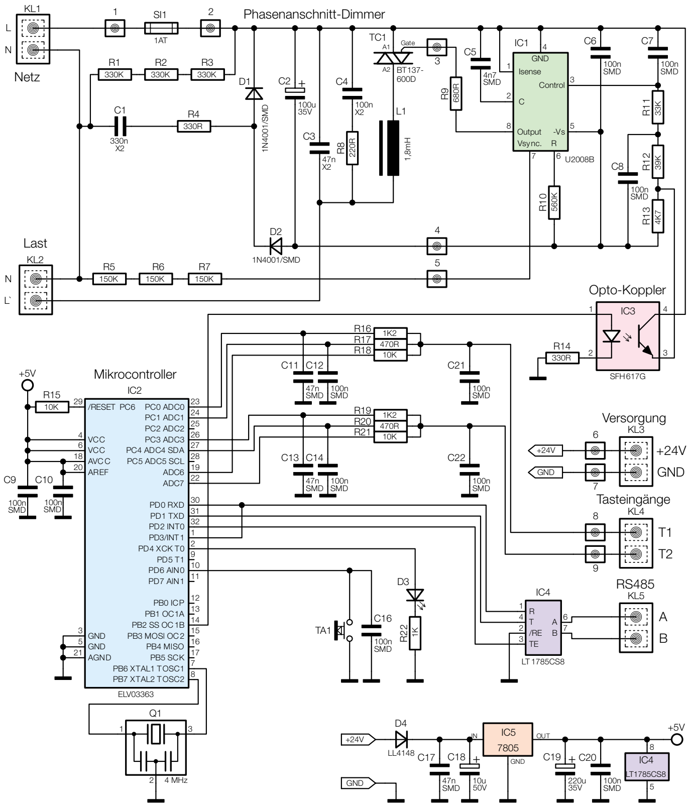
Bild 1: Das Schaltbild des Phasenanschnitt-Dimmers HS485 D
