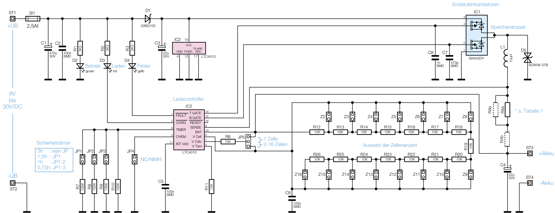
Bild 1: Schaltung des Lade- moduls LM 16
