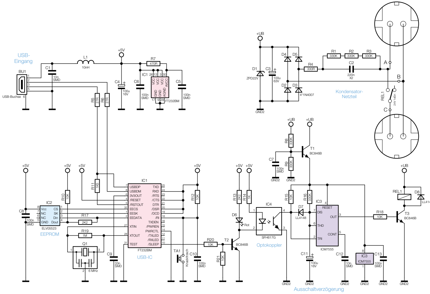
Bild 1: Das Schaltbild des USB-Master-Slave UMS 100
