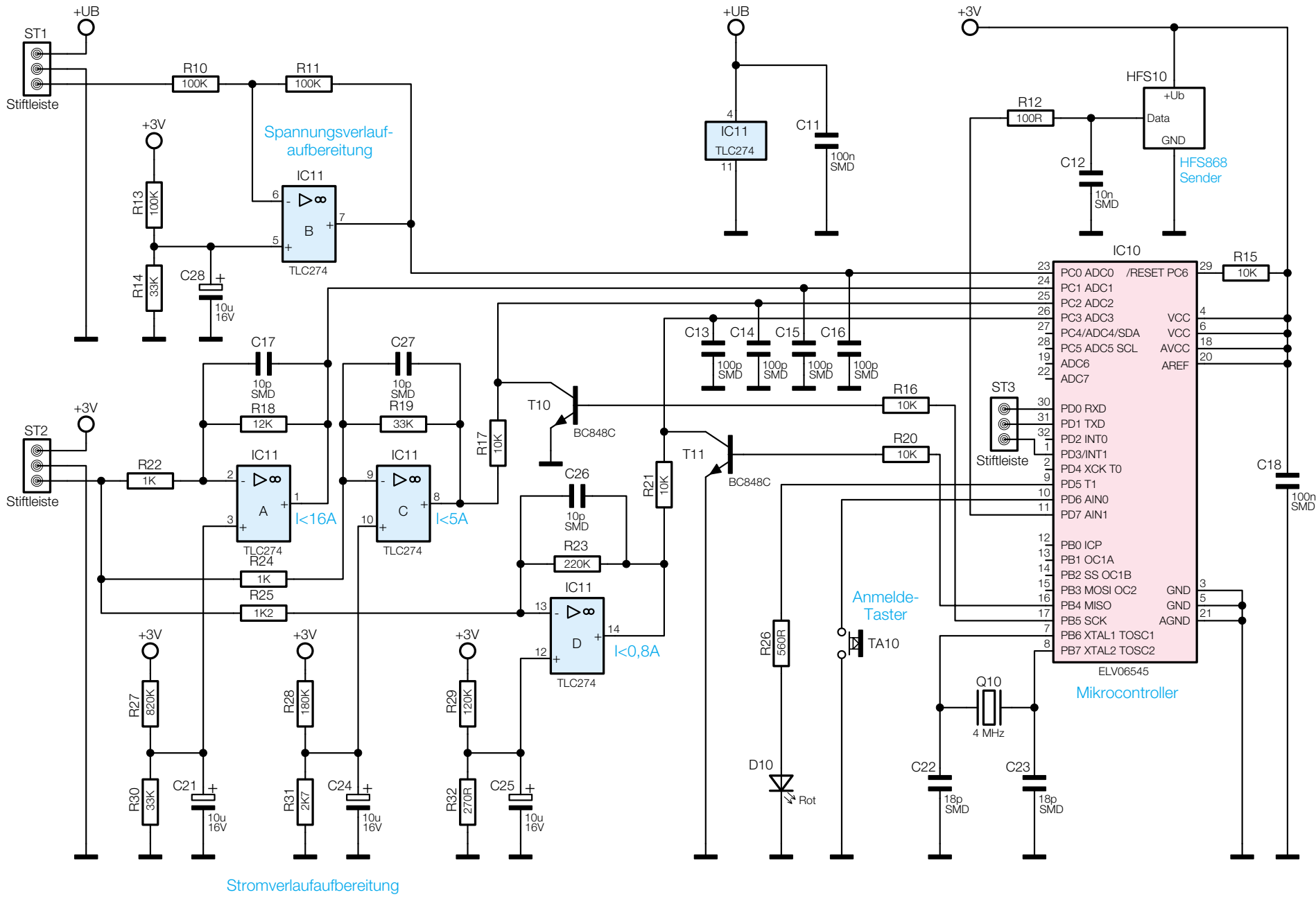
Bild 2: Schaltbild der Steuerplatine des EM 1000-HSM
