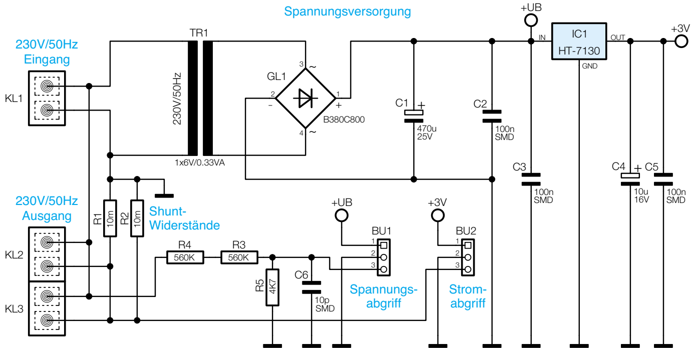
Bild 1: Schaltbild der Basisplatte des EM 1000-HSM
