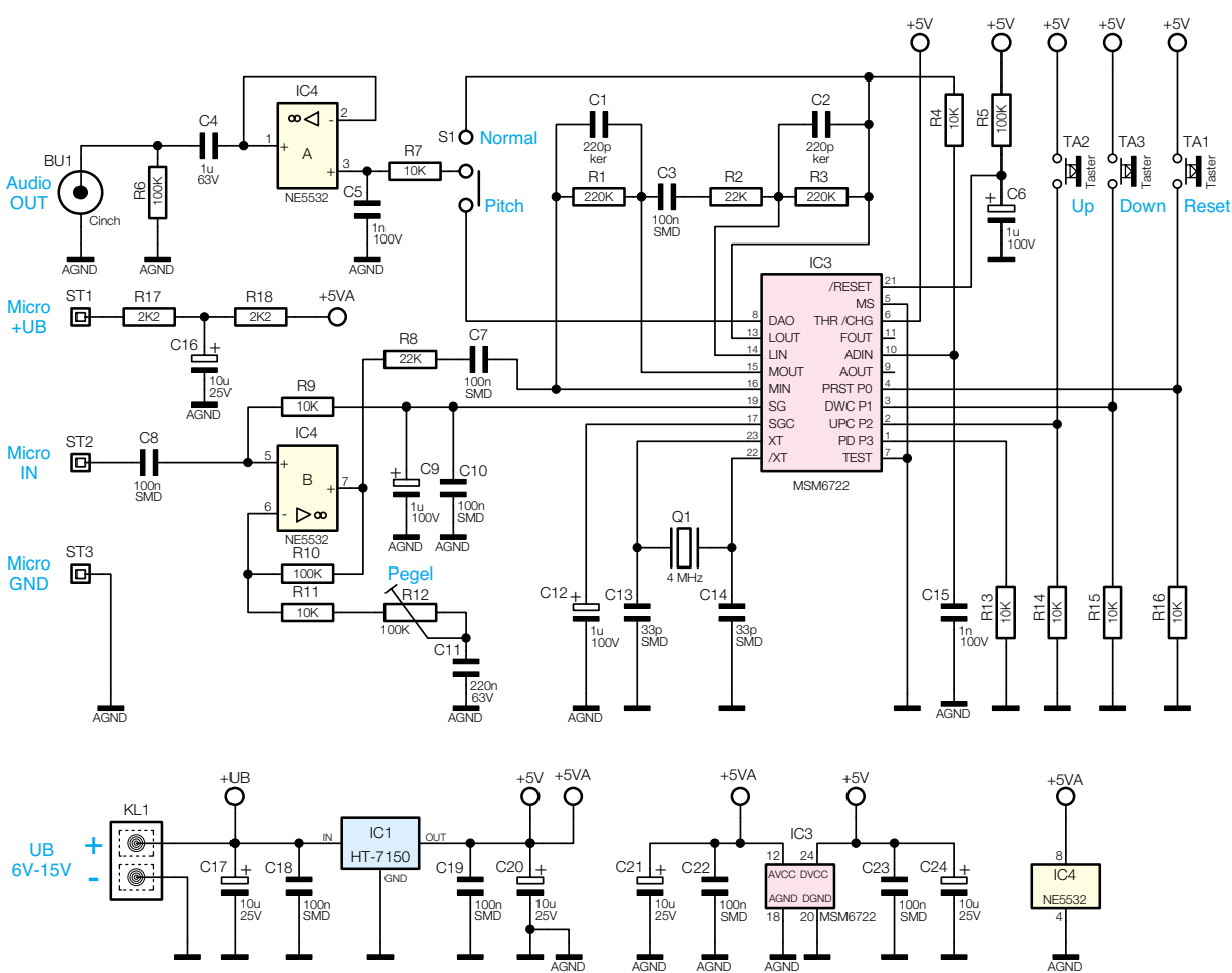
Bild 1: Das Schalt- bild des Voice- Changers
