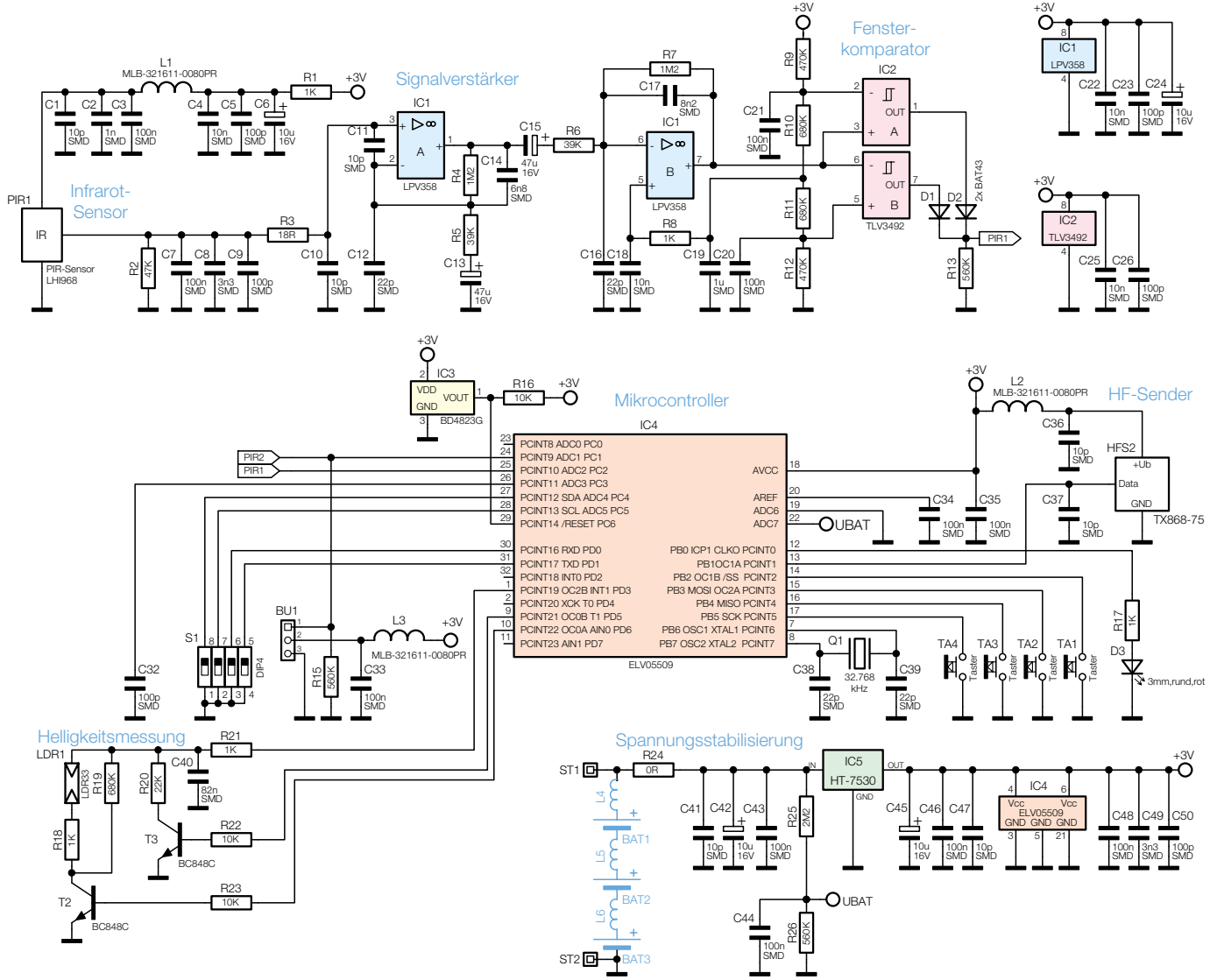
Bild 1: Schaltbild der Hauptplatte
