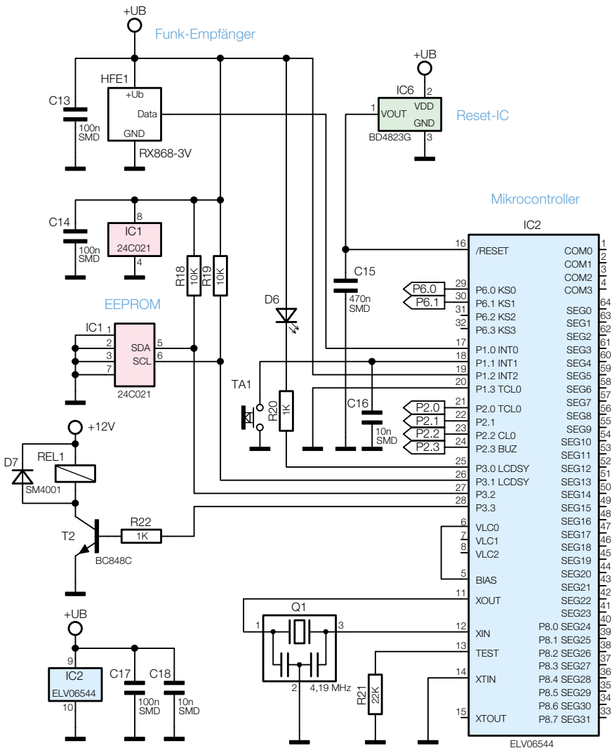
Bild 7: Schaltung des Steuerteils des FS20 DI10
