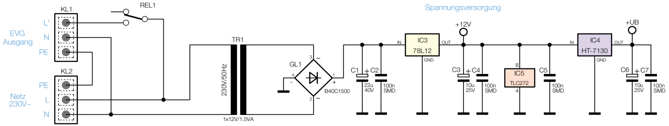
Bild 8: Die Schaltung von Wandler, Verstärkerstufe und Spannungsversorgung des Dimmers
