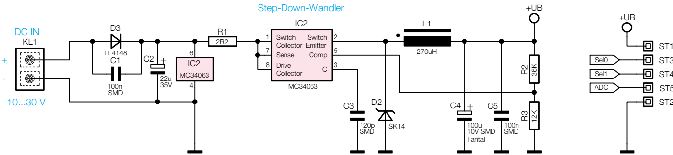
Bild 2: Schaltbild des Prozessorteils und der Spannungsversorgung (Grundplatine)
