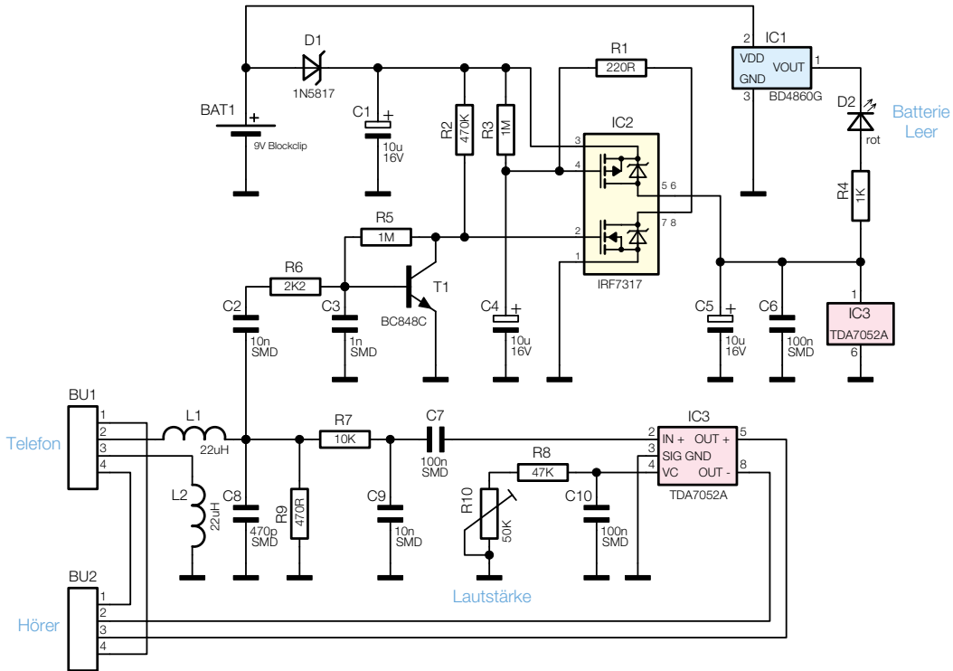
Bild 2: Das Schaltbild des THV 100
