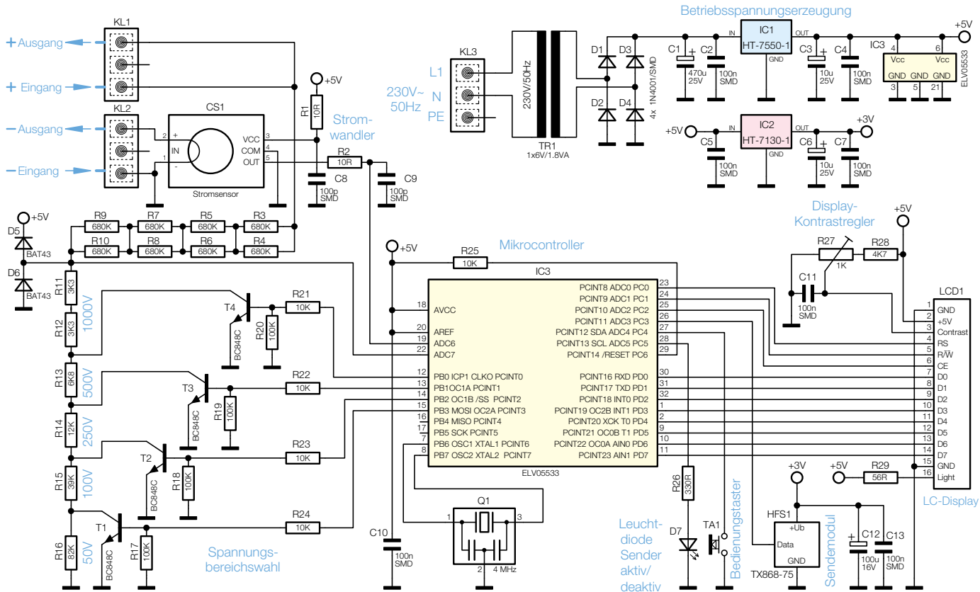
Bild 2: Das Schaltbild des DC-Leistungsmessers.
