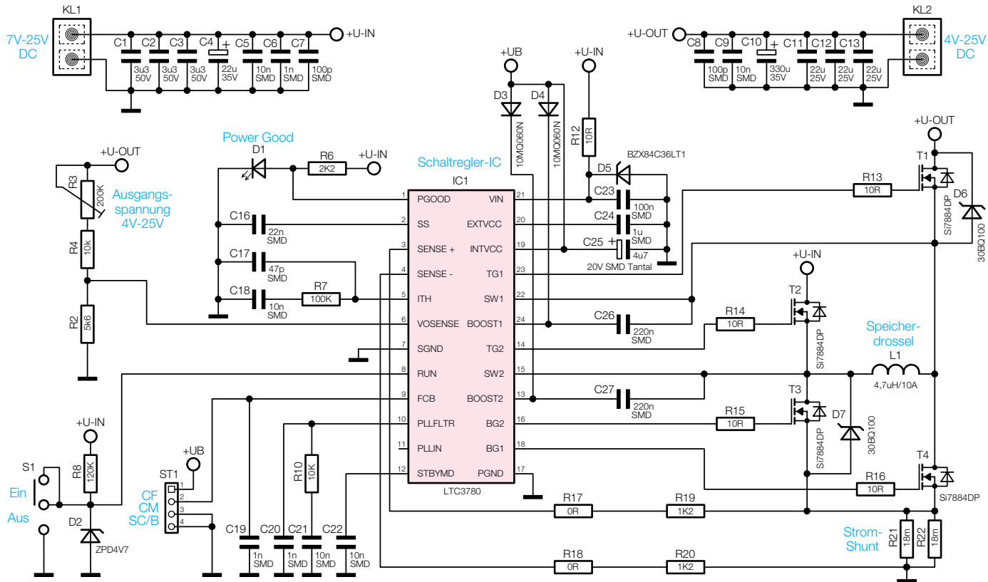
Bild 4: Schaltung des Universal-Spannungswandlers USW 525
