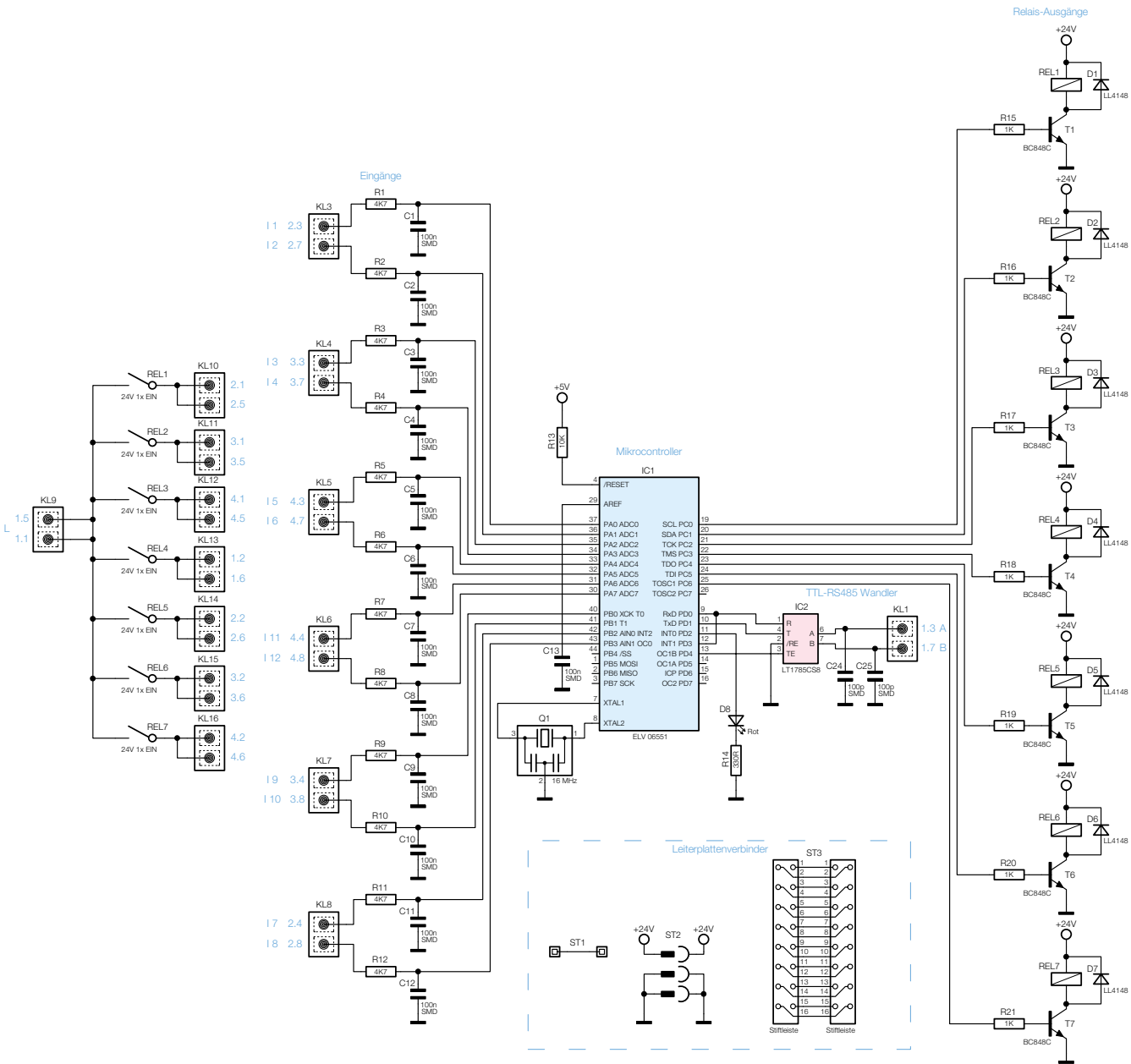
Bild 2: Schaltplan der Mikrocontroller-Steuerung mit Eingangs- und Leistungsteil
