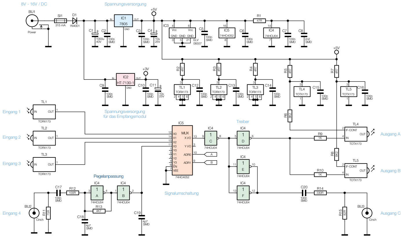
Bild 5: Hauptschaltbild des digitalen Audio-Verteilers DAV 4
