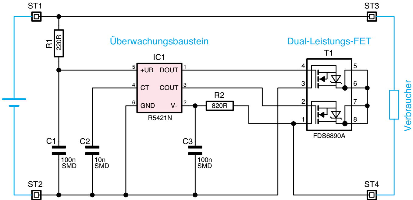
Bild 1: Schaltbild der Lithium-Polymer-Schutzschaltung
