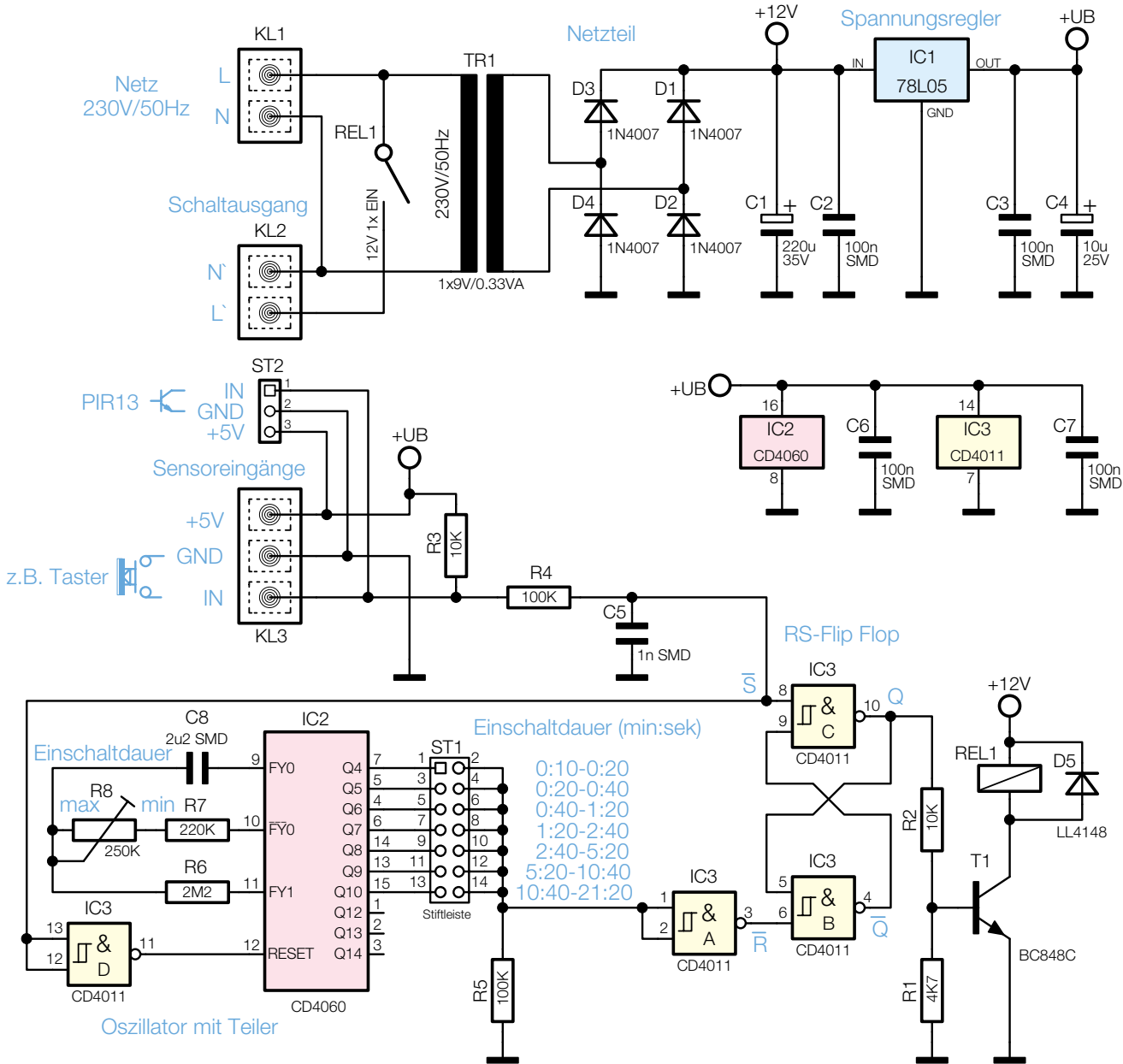
Bild 1: Das Schaltbild des AT 230 ZD
