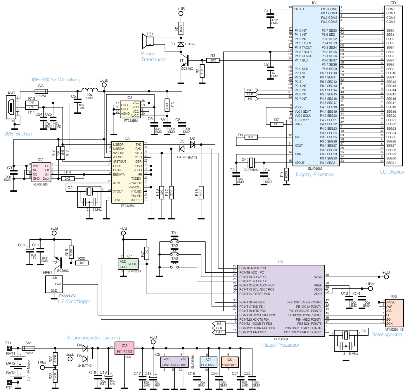
Bild 1: Schaltung des EM 1010 PC
