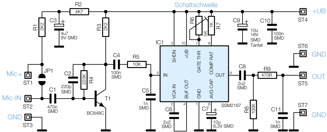
Bild 1: Schaltbild des Mikrofonverstärkers
