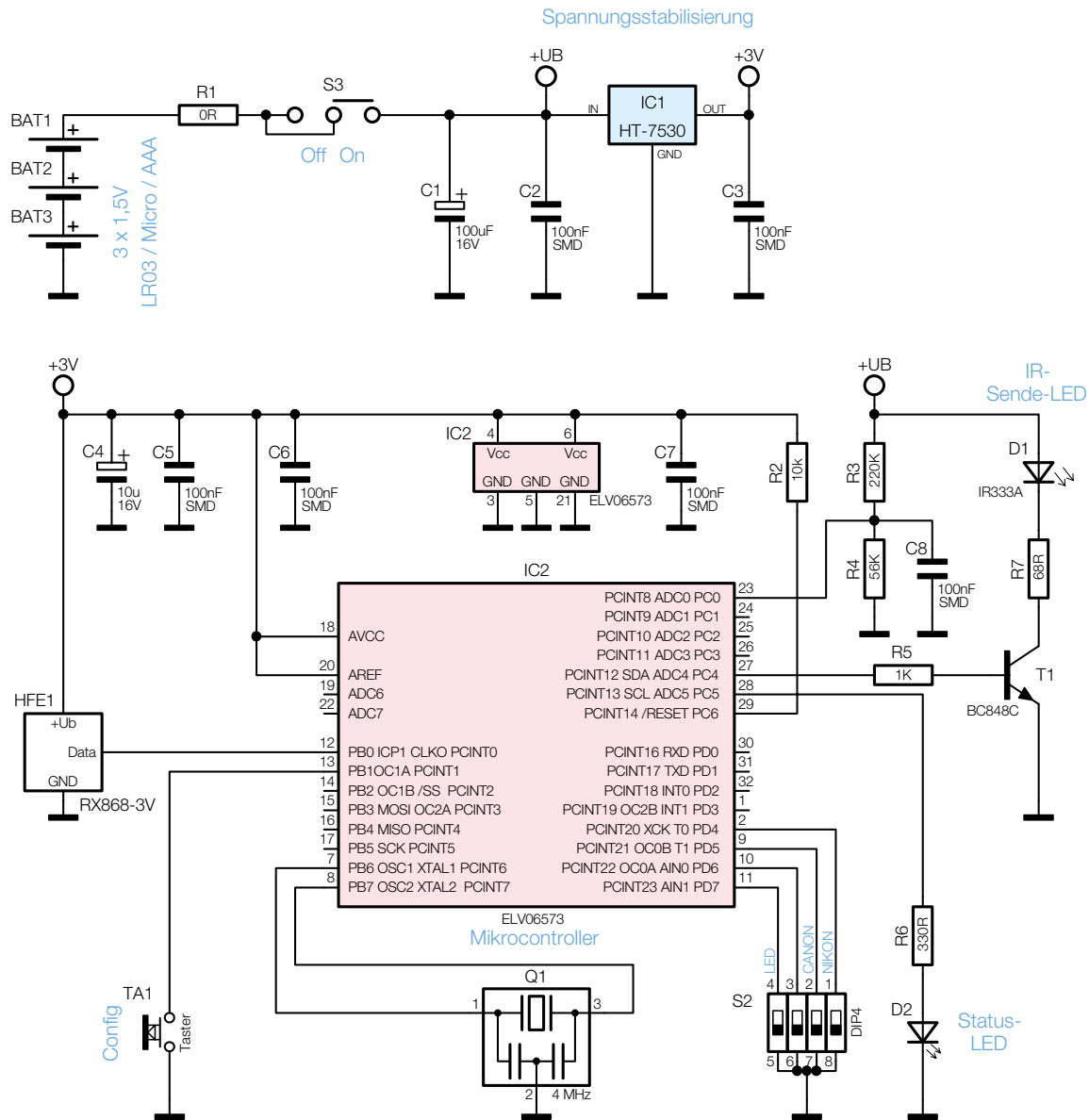
Bild 2: Das Schaltbild des Funk-Fernauslösers
