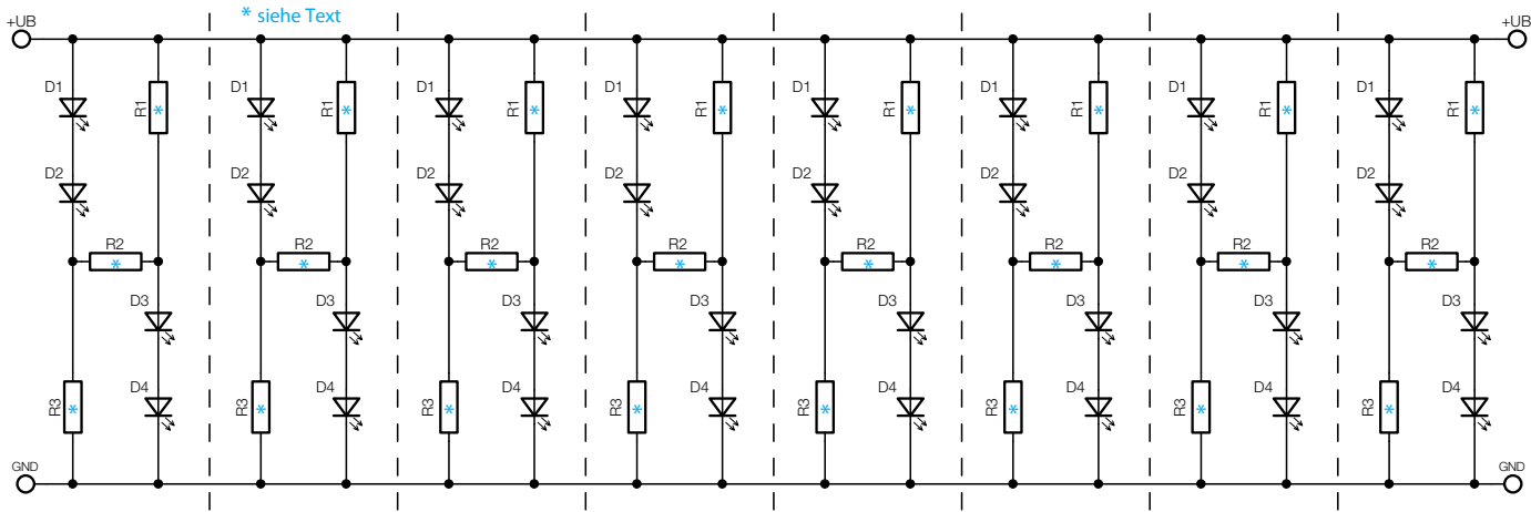
Bild 4: Schaltbild der LED-Stripes 2
