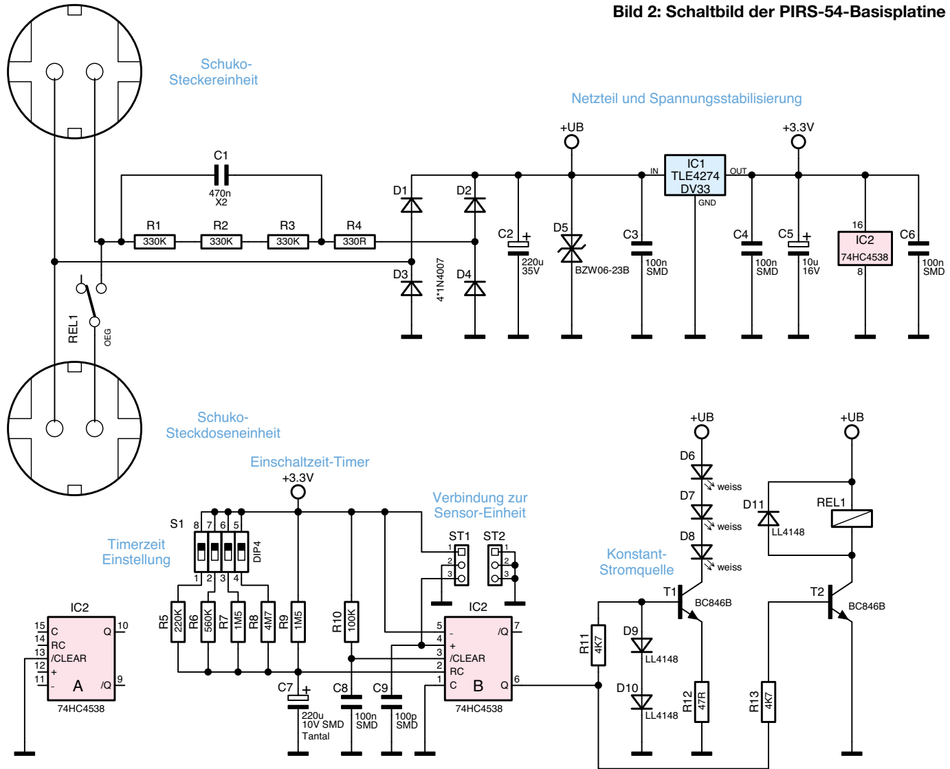
Bild 2: Schaltbild der PIRS-54-Basisplatte
