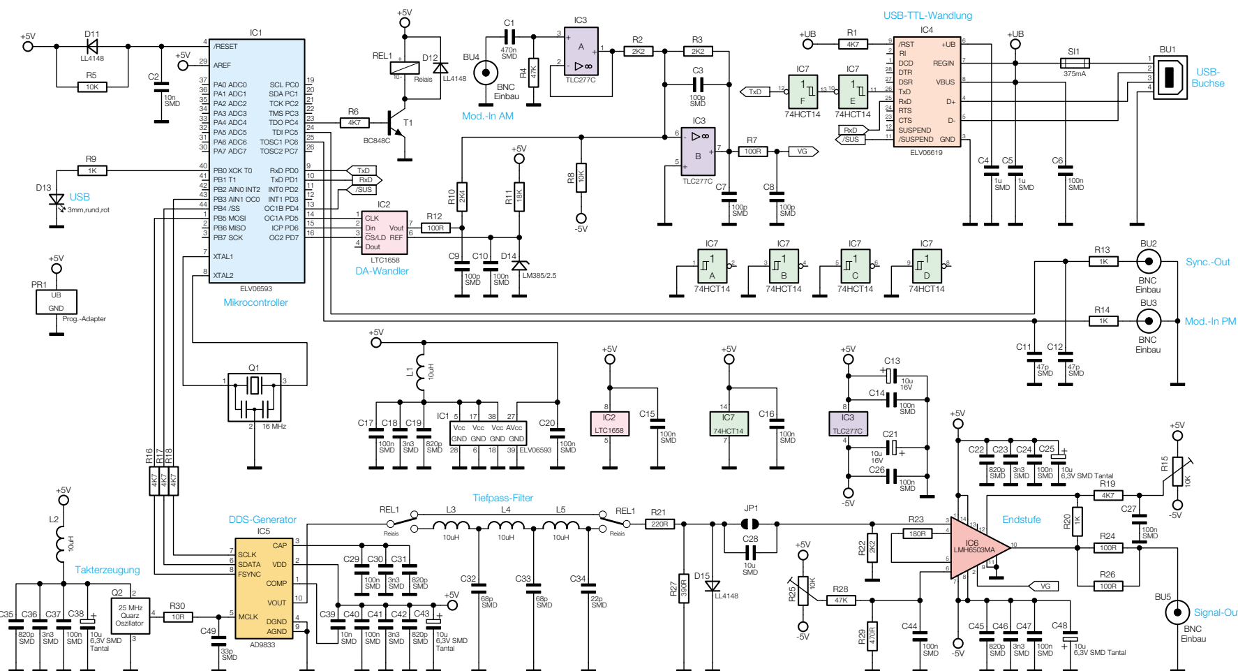
Bild 7: Schaltbild des DDS-Bords
