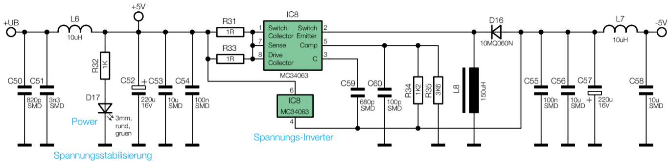
Bild 8: Schaltbild der Spannungsversorgung
