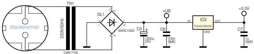
Bild 2: Schaltbild des FS20-Funk-Gongs
