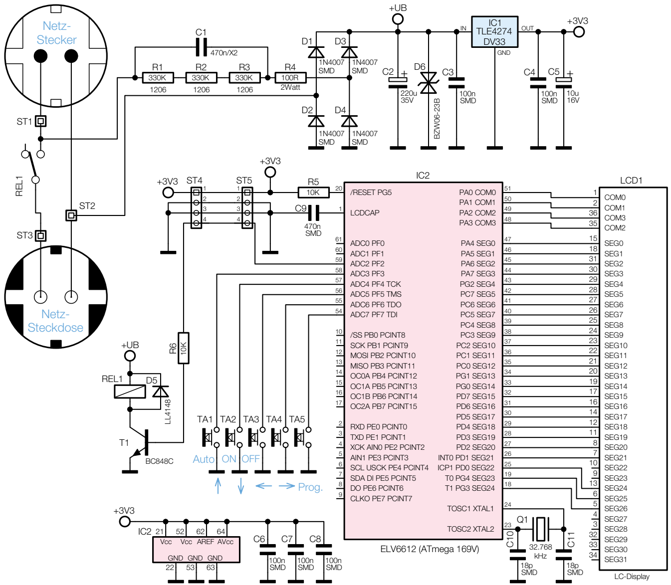
Bild 2: Schaltbild des IVS 53
