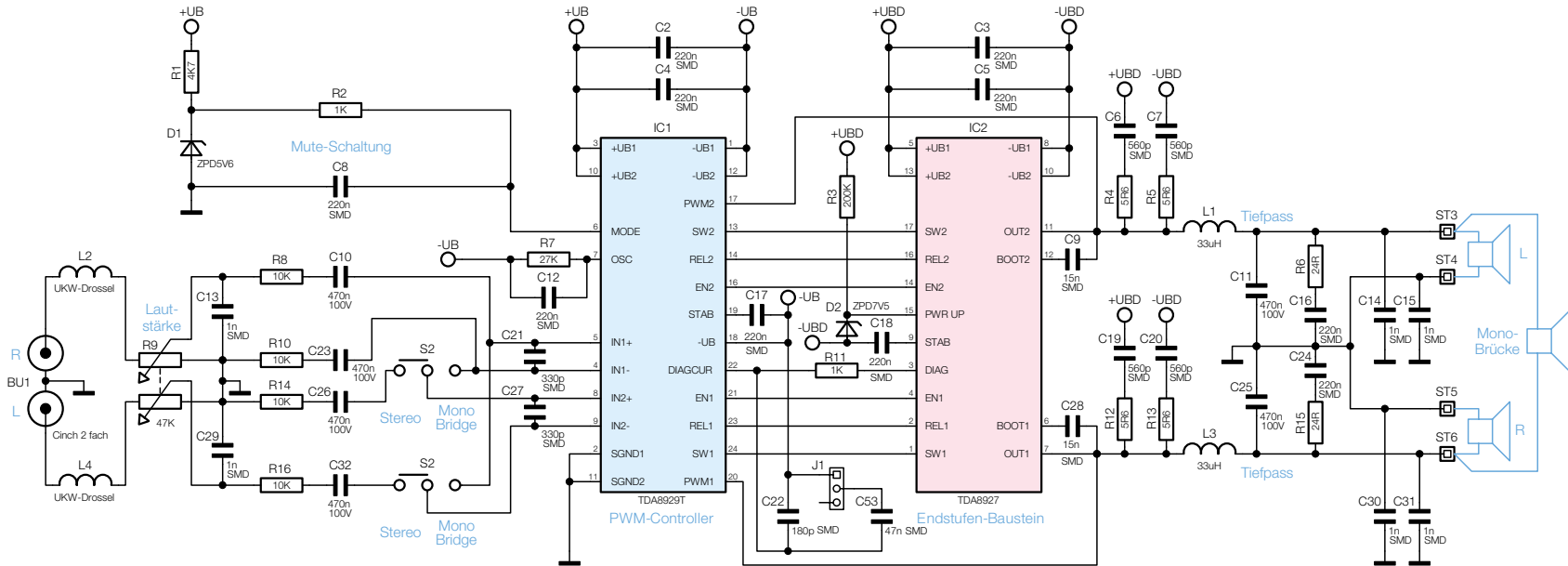
Bild 5: Hauptschaltbild des DA 150
