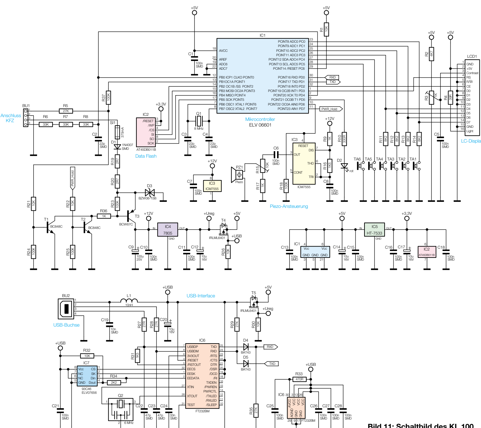
Bild 11: Schaltbild des KL 100
